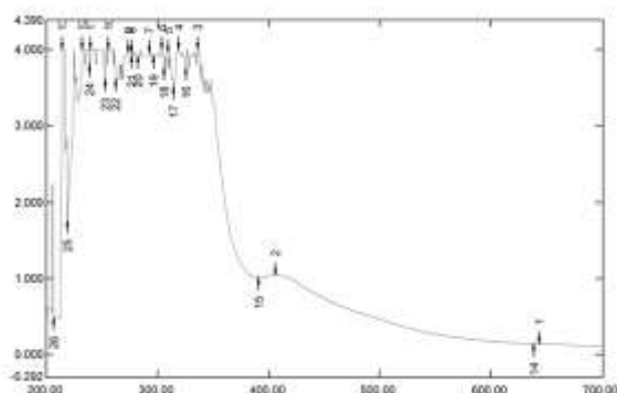
Gambar 1. Spektrum IR ekstrak asam anakardat hasil isolasi menggunakan skema kerja modifikasi.
