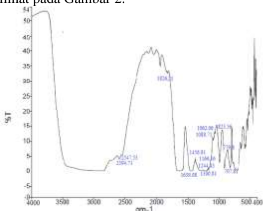
Gambar 1. Spektrum IR ekstrak asam anakardat hasil isolasi menggunakan skema kerja modifikasi.
