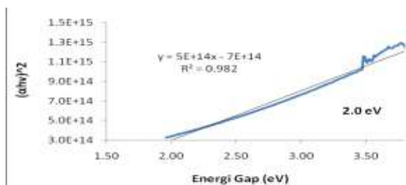
Gambar 6. Grafik (\alpha h\nu)^2 sebagai fungsi energi gap lapisan tipis ZnO suhu 400 °C pada 1,0M
